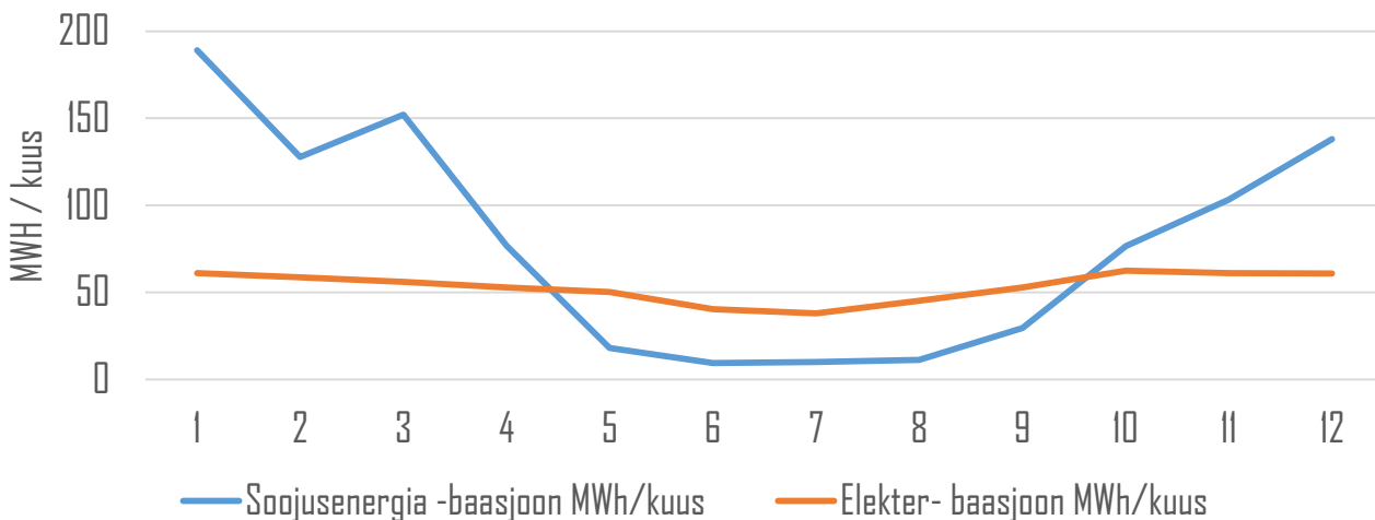
Energiatarbimise profiil
