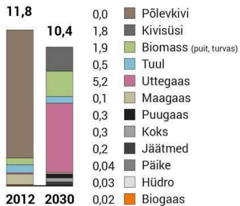
2012 2030 Elektritootmine, TWh
