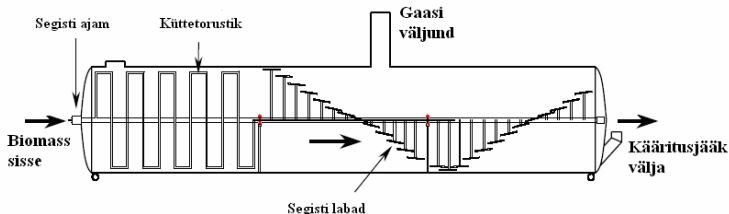
Joonis 5. Rõhtne kääríti [5].
