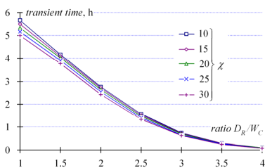
Joonis 9. Teoreetiliselt arvatud varjusiire sisemisel moodulil.
