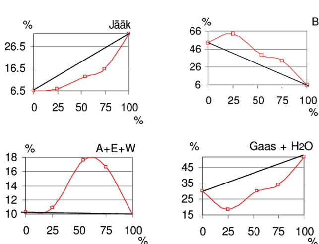
Joonis 3. Vesikonversioonisaaduste saagised vastandatuna aditiivsele saagisele (must sirge joon) % OA-st (tähised vt jn 1)
